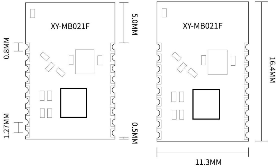
图 2-模块尺寸图
