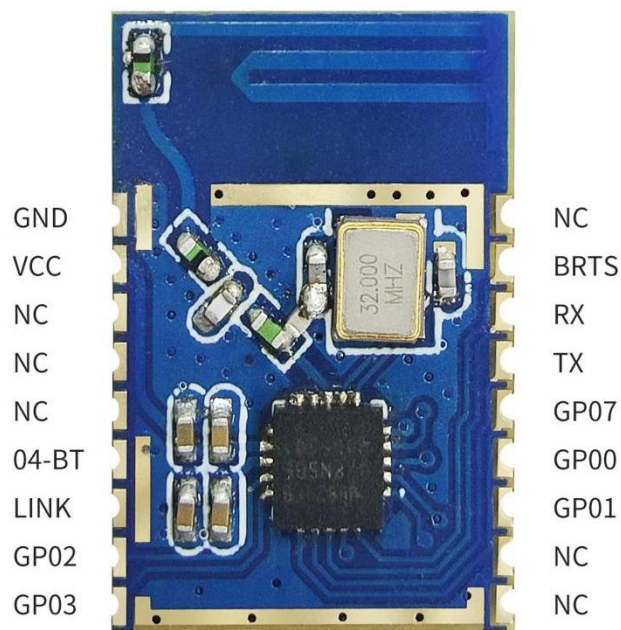
图 1-模块引脚图
