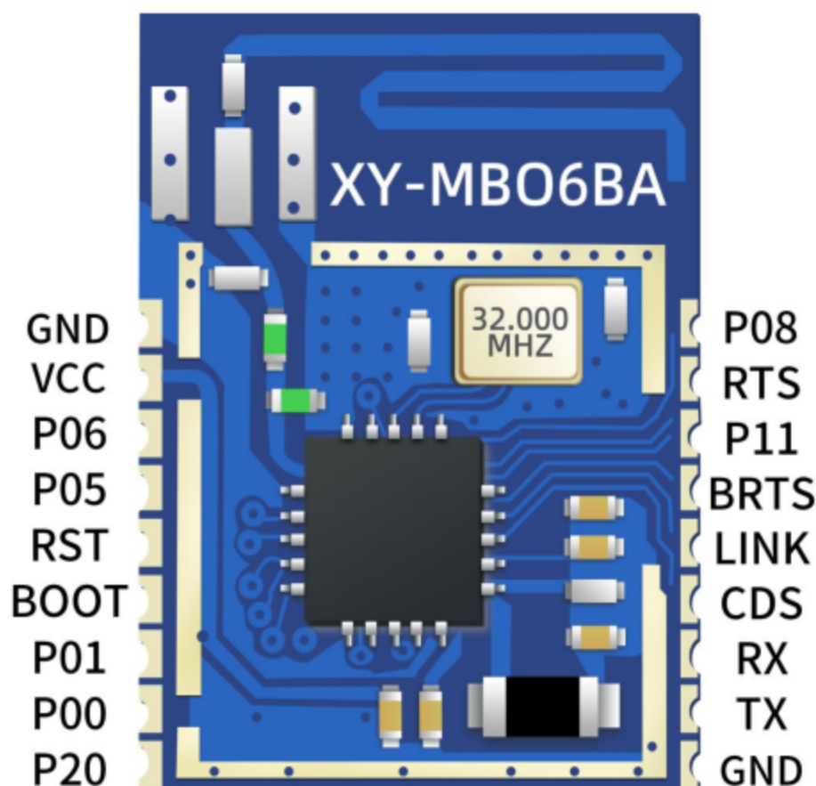
图 1-模块引脚图
